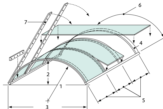
1 = Radius 4 = Bügel 6 = Bogenlänge 2 = Stichhöhe 5 = Bügelabstand 7 = Deckleiste 3 = Spannweite
