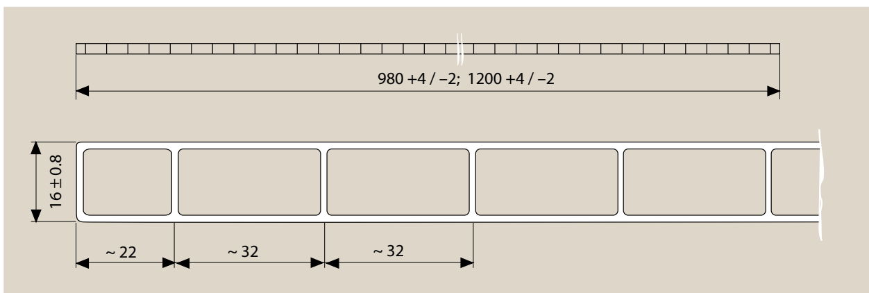
Querschnittsbild der PLEXIGLAS HEATSTOP® Opal SDP 16 (Maße in mm)
