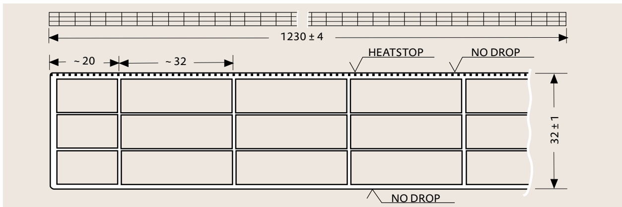
Querschnittbild der PLEXIGLAS HEATSTOP® Transparent S4P 32 (Maße in mm)
